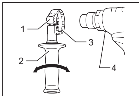
► 1. Grip base 2. Side grip 3. Teeth 4. Protrusion
