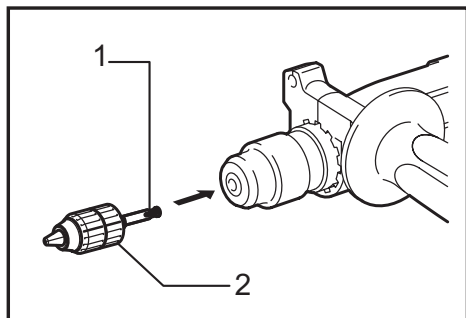
► 1. Adaptador de mandril 2. Mandril sin llave
